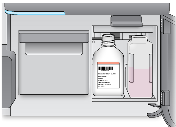
Figur 12 Sett inn flasken med MiSeqDx SBS Solution (PR2).
