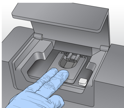
Figur 11 Lukke strømningscellesperren
