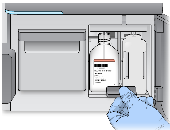
Figur 13 Senke sugeenhetshåndtaket
